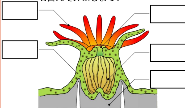
ポリプ (サンゴ個体)
